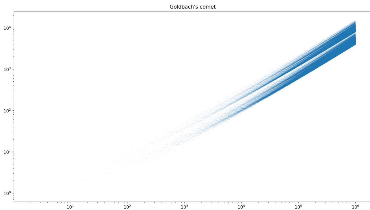
Comète de Goldbach : déformation logarithmique sur les deux coordonnées (jusqu'à 10^6 ).
