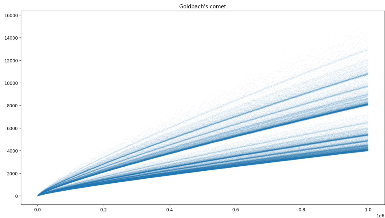
Comète de Goldbach : en abscisse les nombres pairs, en ordonnée leur nombre de décompositions de Goldbach.
