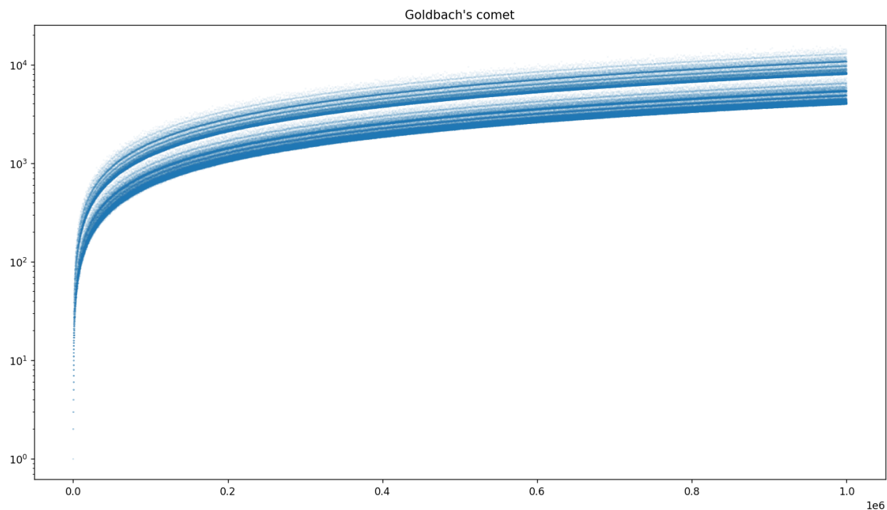
Comète de Goldbach : déformation logarithmique sur l'ordonnée.
