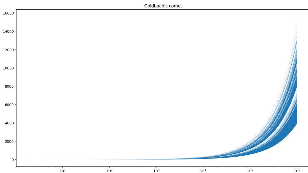
Comète de Goldbach : déformation logarithmique sur l'abscisse.
